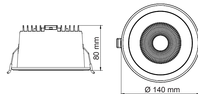
Dimensions
