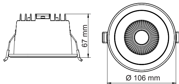
Dimensions
